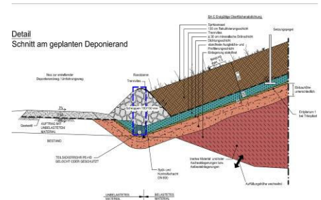
Systemaufbau Oberflächenabdichtung
